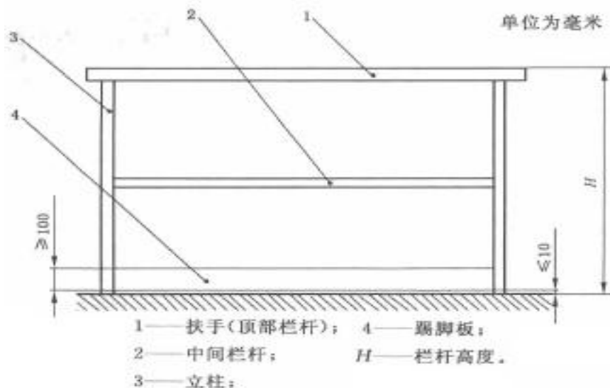
图 1 防护栏杆示意图
